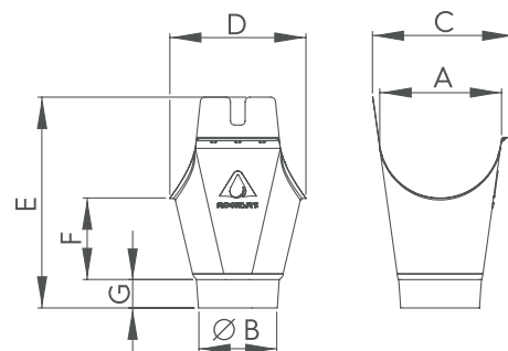
Dimensiuni element (mm)
