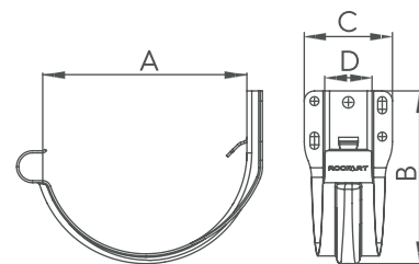
Dimensiuni element (mm)
